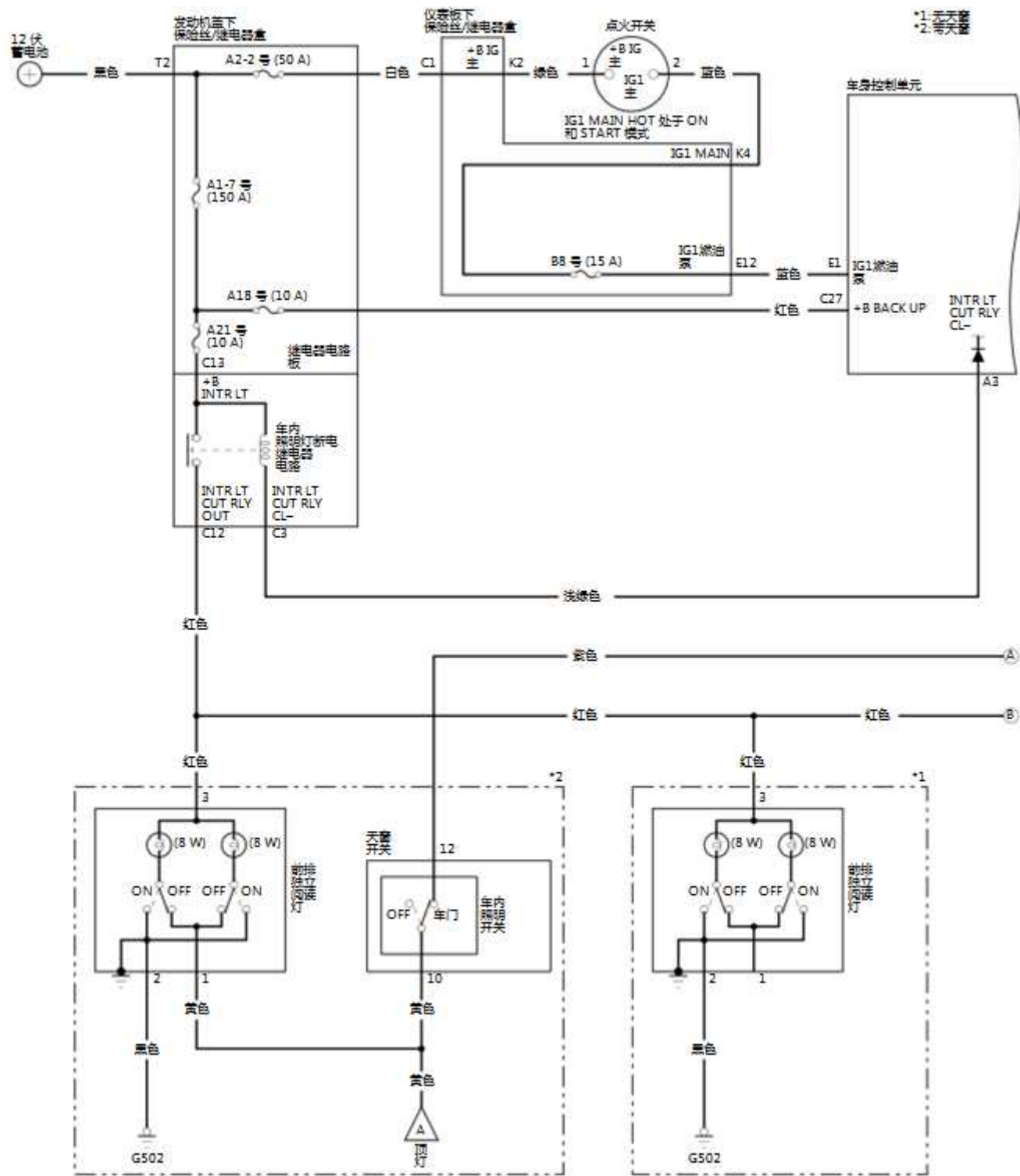
车内照明灯电路图
